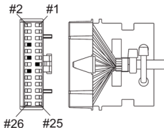
Abbildung 1. 26-poliger Blockstecker
