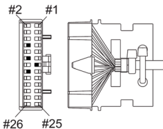
Figura 1. Bloque de conexión de 26 pines
