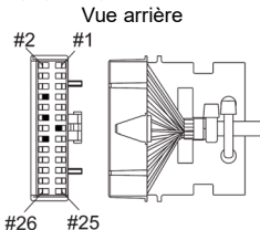
Figure 1. Bloc de connexion 26 broches
