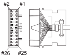
Afbeelding 1. 26-polige blokstekker
