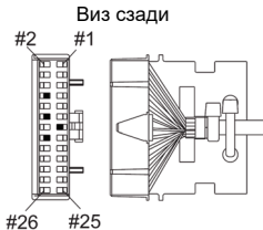
Рис. 1. 26-штырьковый разъем
