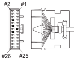
Figura 1. Bassetta connessioni a 26 pin
